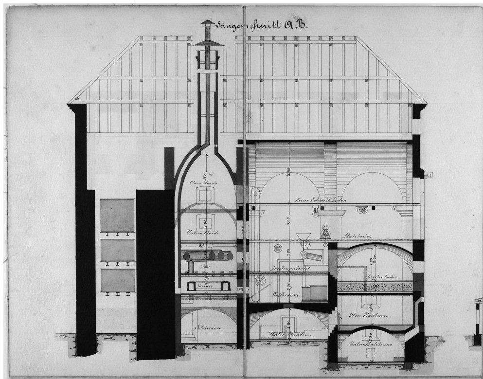
Aufriss des Bräuhauses in der ehemaligen Stiftskirche Herrenchiemsee
