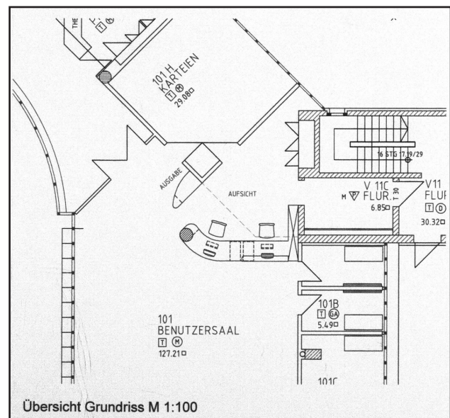
Abb. 2: Neue Theke – Planung des Staatlichen Bauamtes Augsburg (Frühjahr 2011)
