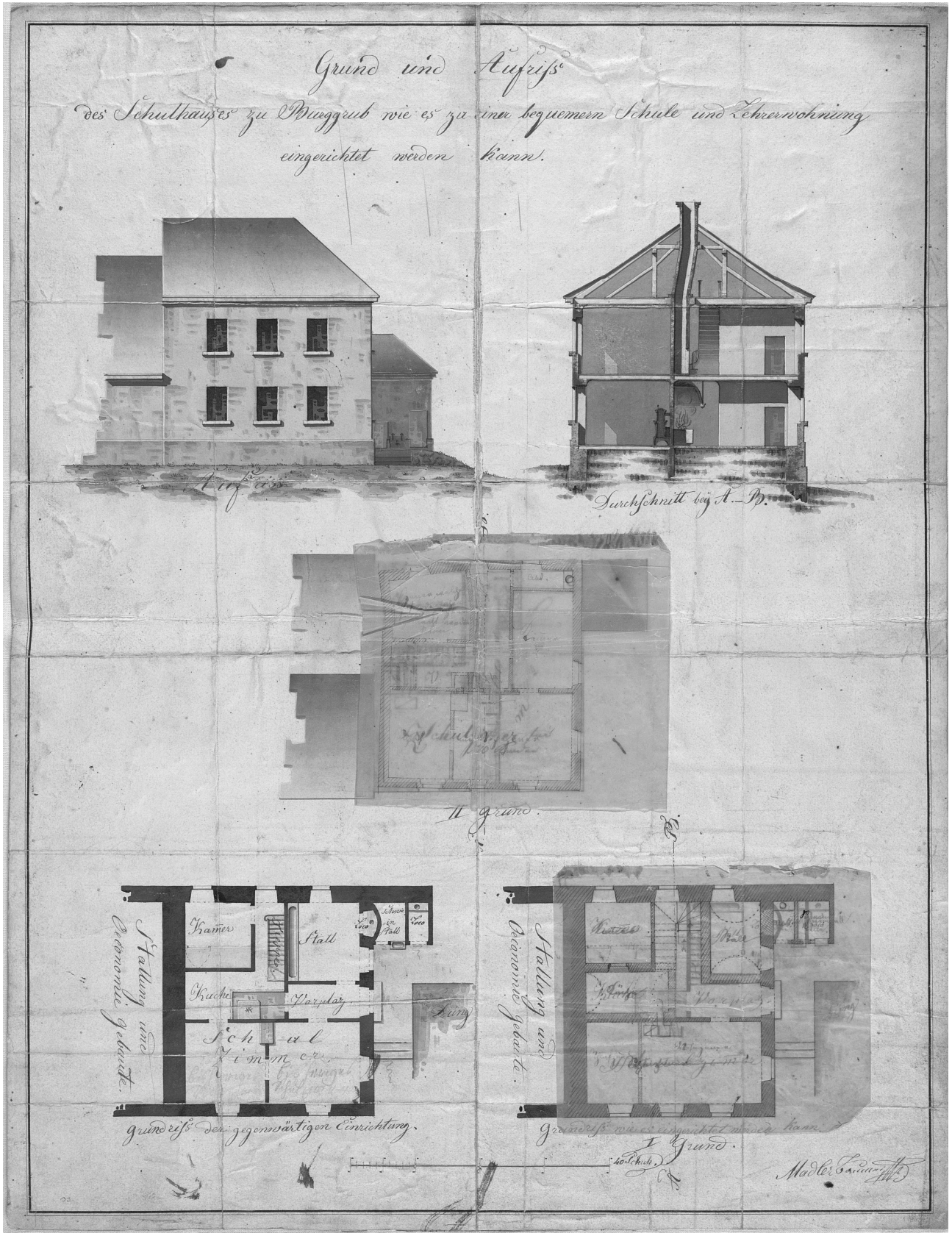
Grund- und Aufriss des Schulhauses in Burggrub mit Überlegungen zu Umbaumaßnahmen, Anfang 20. Jahrhundert (Staatsarchiv Bamberg, Schenk v. Stauffenberg zu Greifenstein Nr. 2108) (Foto: Staatsarchiv Bamberg)
