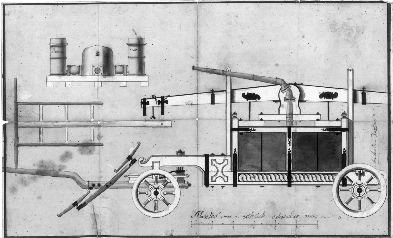
Plan einer neuen Feuerspritze für die Stadt Burghausen von 1799, Entwurf des Stuck- und Glockengießers Johann Georg Stecher (Staatsarchiv München, Regierung Burghausen 4148) (Foto: Bayerisches Hauptstaatsarchiv)
