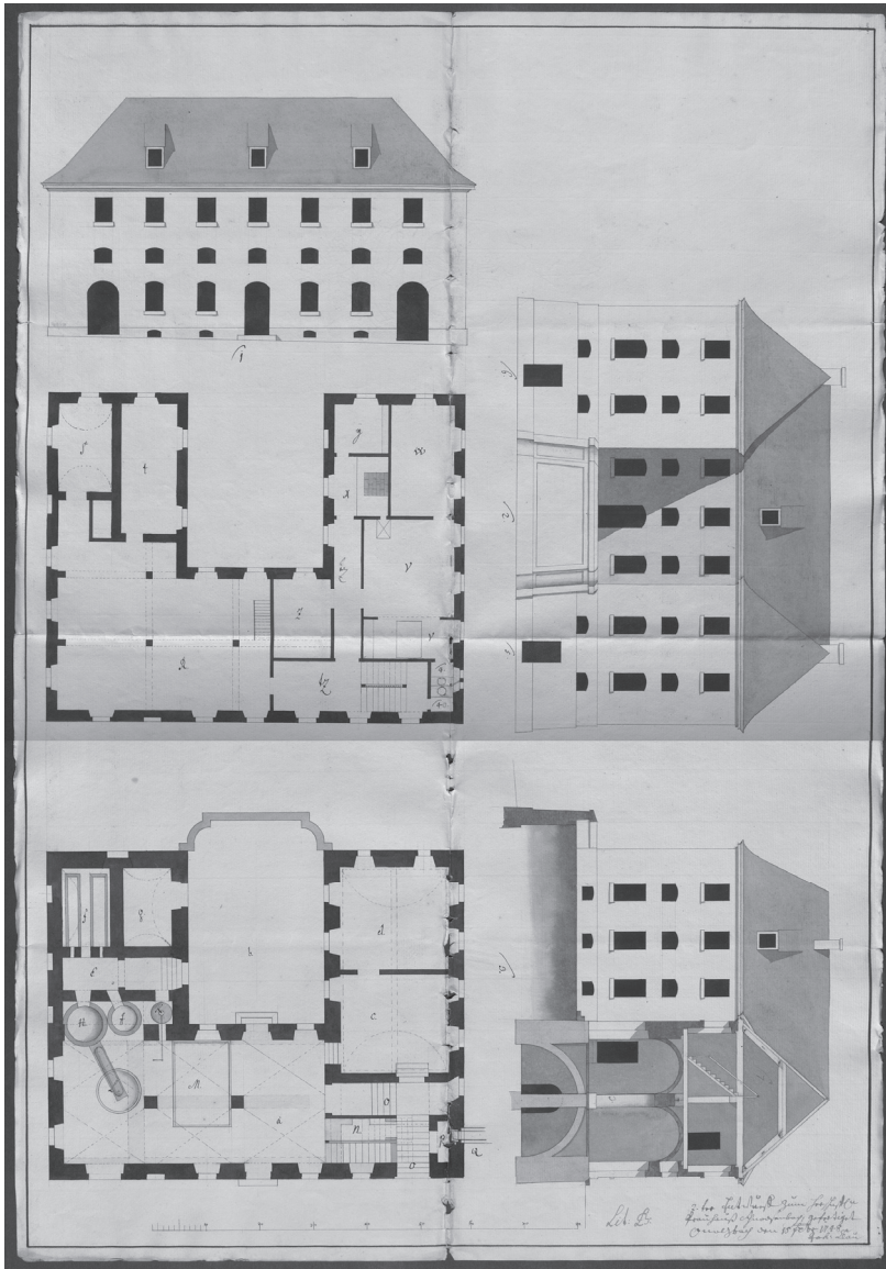
Entwurf für ein schlossartiges Brauhaus zu Schnodsenbach von dem Ansbacher Hofmaurer Johann Clau 1748 (Staatsarchiv Nürnberg, Gefürstete Grafschaft Schwarzenberg, Schnodsenbach Nr. 31/24, Prod. 42) (Foto: Klaus Drechsler, Staatsarchiv Nürnberg)
