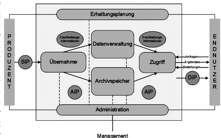
Grafische Darstellung des OAIS-Modells (Quelle: nestor – Kompetenznetzwerk Langzeitarchivierung: nestor-materialien 16 – Referenzmodell für ein Offenes Archiv- Informations-System – Deutsche Übersetzung, Version 2.0, Frankfurt am Main 2013, S. 33)
