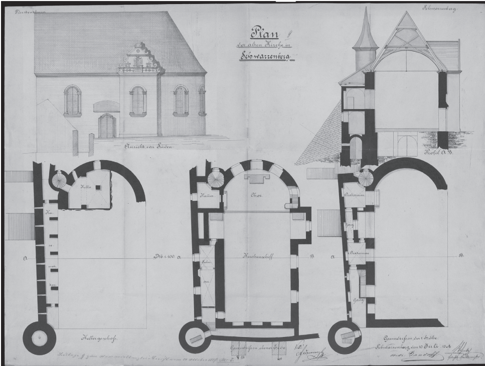
Plan der Kapelle des Schlosses Schwarzenberg anlässlich der Renovierungsarbeiten, Maßstab 1:100, gezeichnet W. Hinke 1888 (Staatsarchiv Nürnberg, Herrschaft Schwarzenberg, Karten und Pläne Nr. 11, Provenienz: Bauverwaltung) (Foto: Klaus Drechsler, Staatsarchiv Nürnberg).
