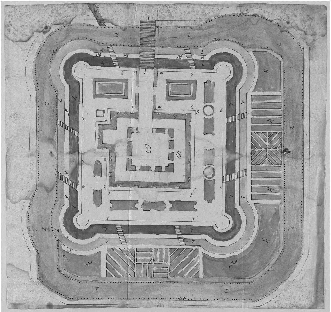
Plan von Schloss Gebelkofen, 1779 (Schlossarchiv Köfering vorl. Nr. 330) (Foto: Staatsarchiv Amberg).
